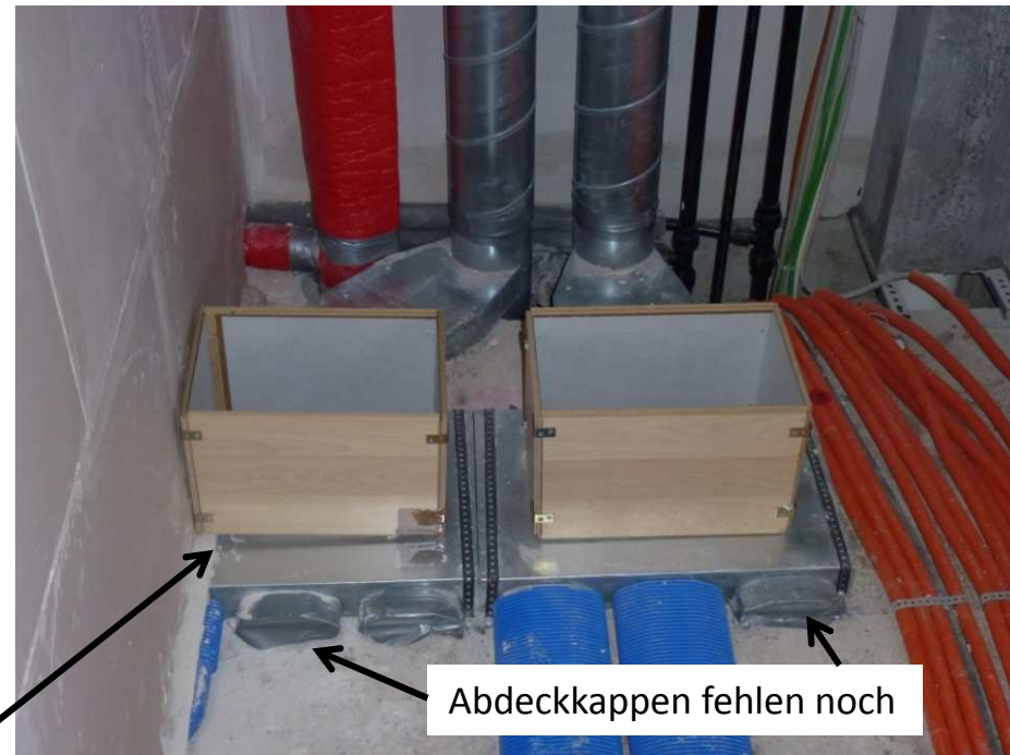
Bastellösung: Zugang zu den Reinigungsöffnungen
